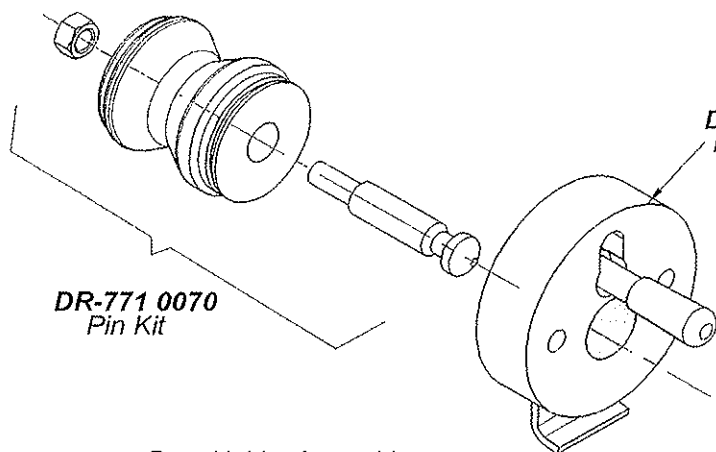
Door Holder Assembly
